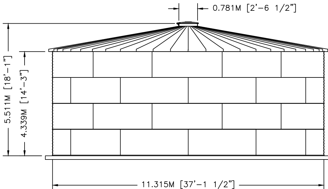
ELEVATION
