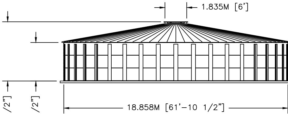
ELEVATION
